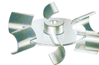
HY型六圆弧叶圆盘涡轮式 HY type
